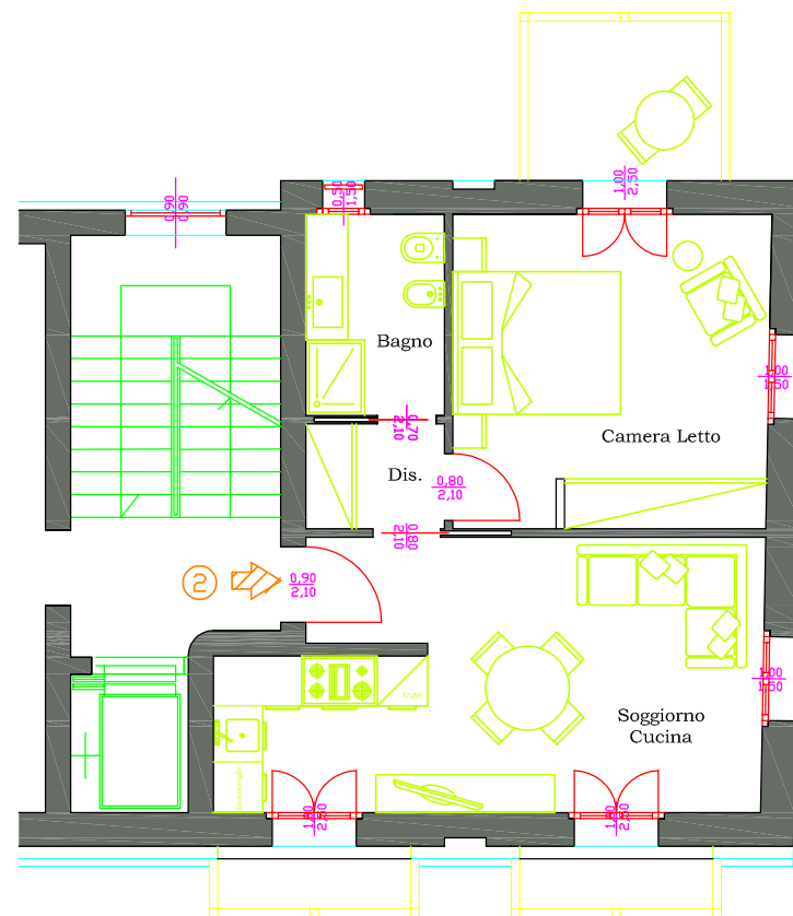
PIANO PRIMO
