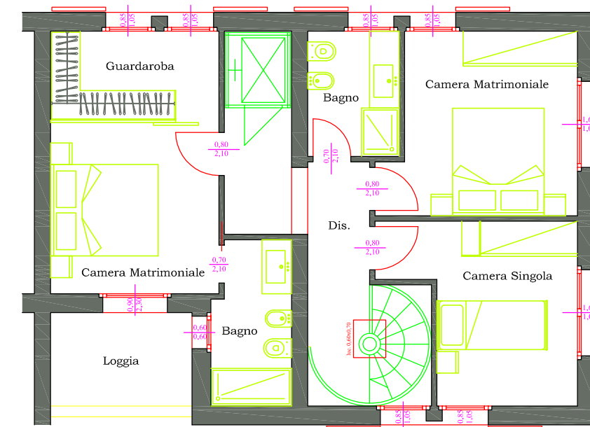
PIANO PRIMO
