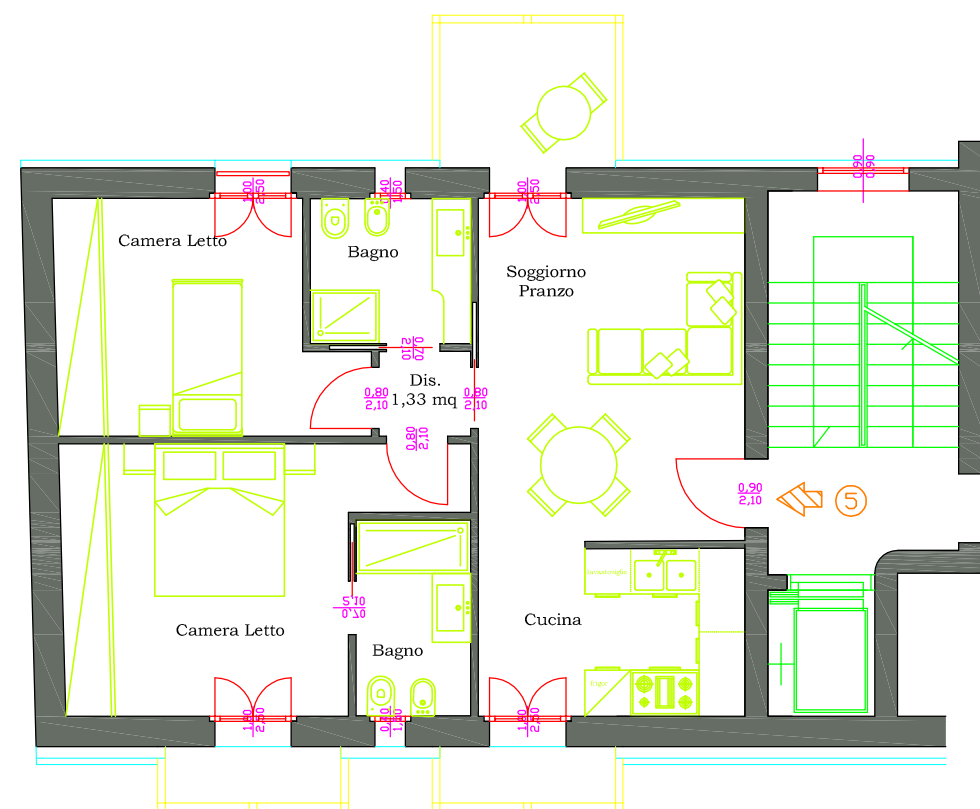
PIANO TERZO
