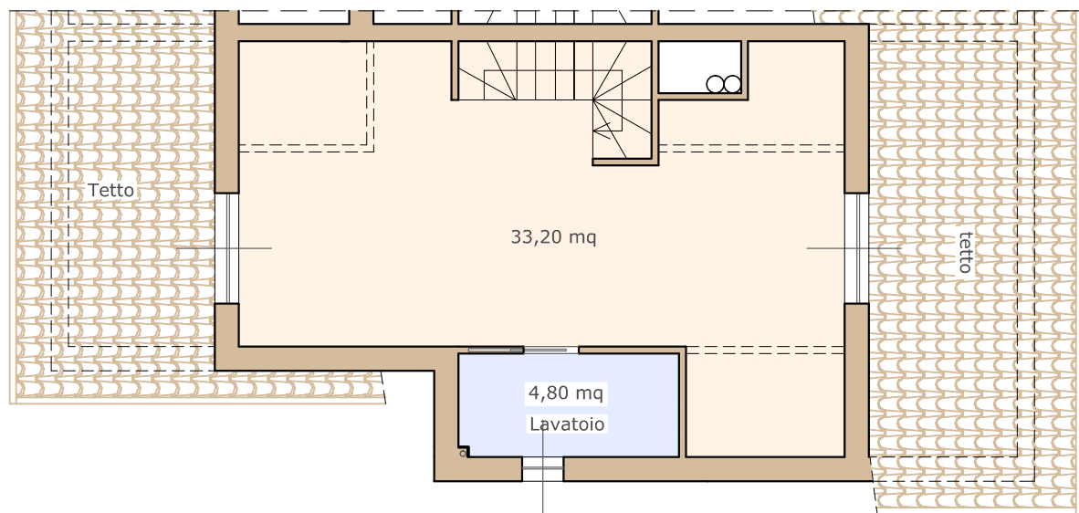
Pianta piano primo 1:100
