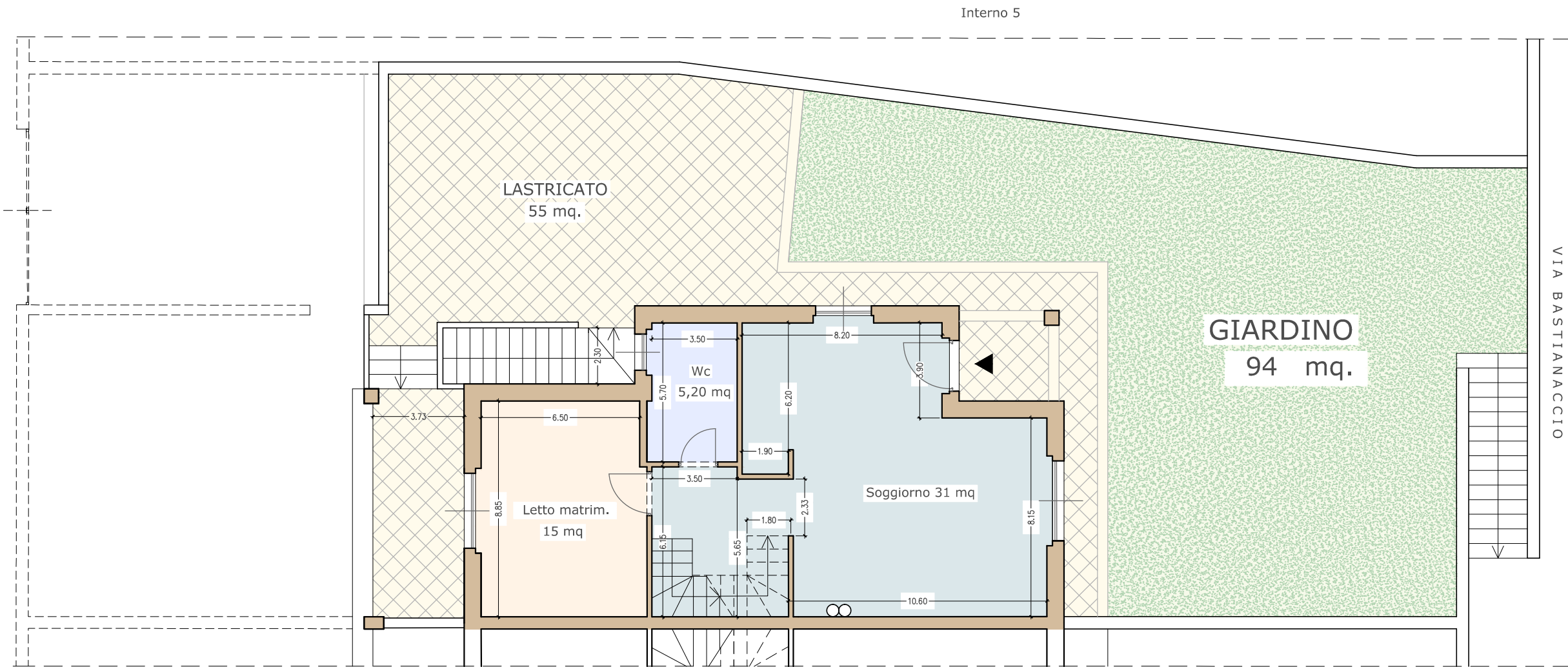
Pianta piano terra 1:100
